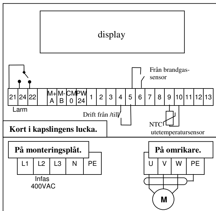
Figur 2. Inkoppling för tryckreglering med temperaturkompensering med fast frekvens aktiverad från brandgas-sensor på en FKP-X 400V drift.
