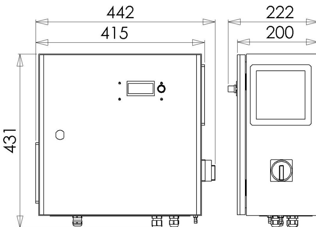
Figur 11. FKP-X 400V dimensioner. Visar här de minsta dimensionerna. FKP-X i höga effekter och varm omgivning kan behöva kapslas i större kapsling för att öka ventilationen.
