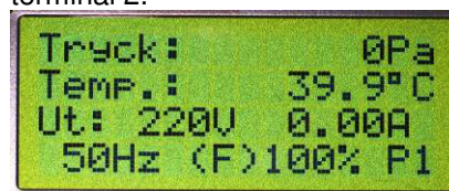
Figur 10. FKP-X informationsskärm i tryckreglerat läge med utetemperaturkompensering och aktivt veckoschema där program P1 körs med 100% av tryckbörvärdet. F:et visar att driften går i forcerat läge.
