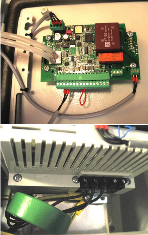
Figur 3. Elektrisk och mekanisk inkoppling av FKP-X i normal fläktapplikation med ferritring på utgående motorfaser. Byglad för rotationsriktning framåt och uttemperatursensor på terminal 9,10. Se Inkoppling för beskrivning av inkoppling av motorkabel.
