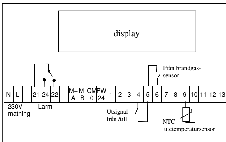
Figur 1. Inkoppling för tryckreglering med temperaturkompensering med fast utsignal aktiverad från brandgas-sensor. Utetemperatursensor på terminal 9,10.
